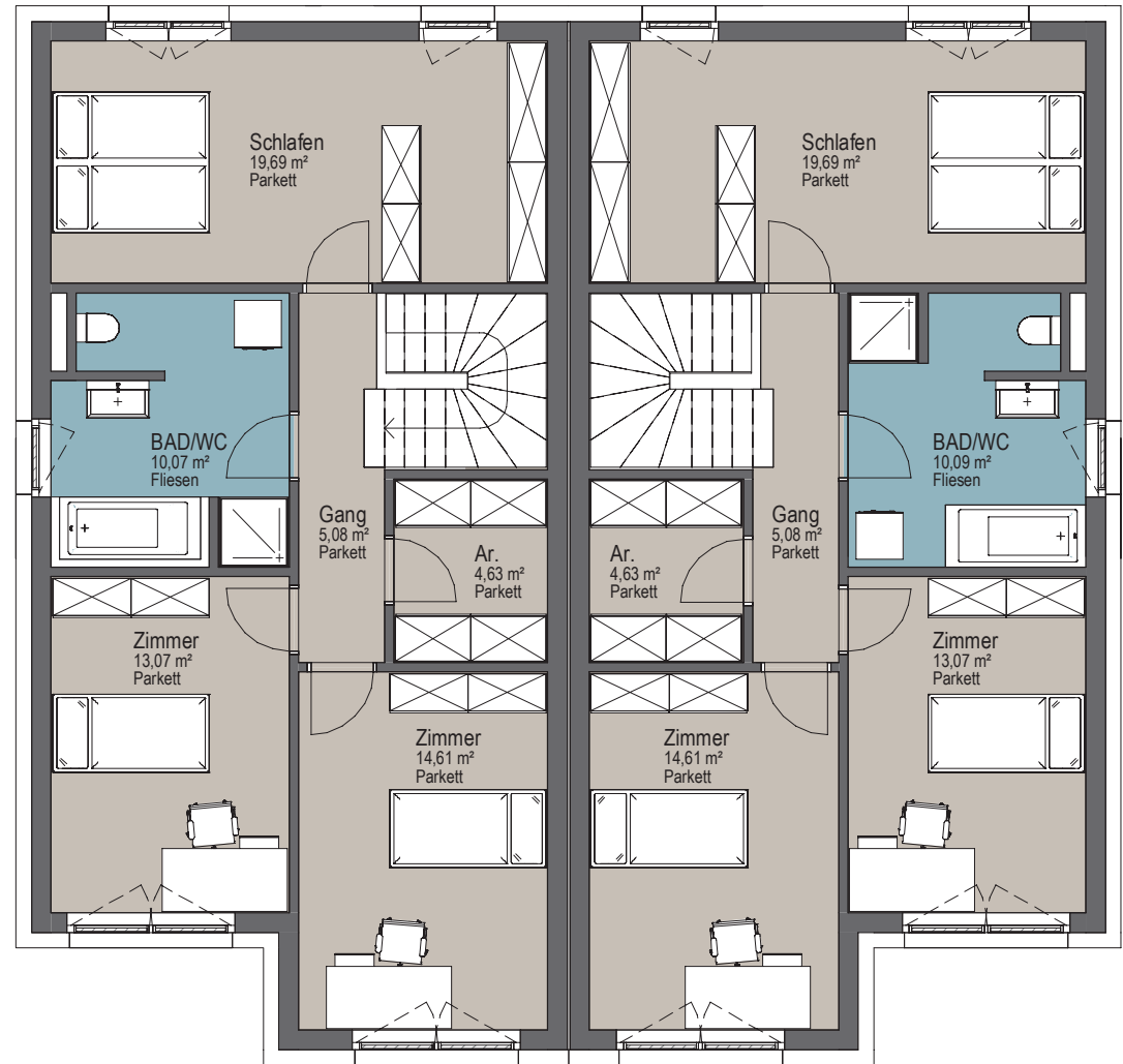
OBERGESCHOSS
