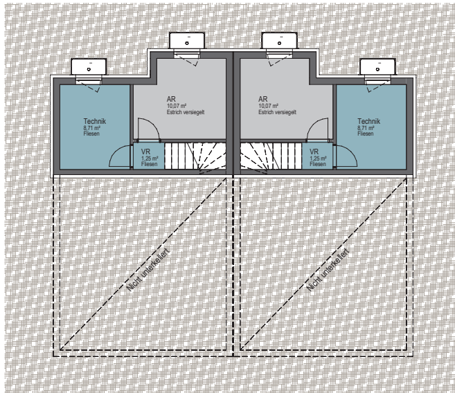
UNTERGESCHOSS PLANSTAND 27.04.2020
