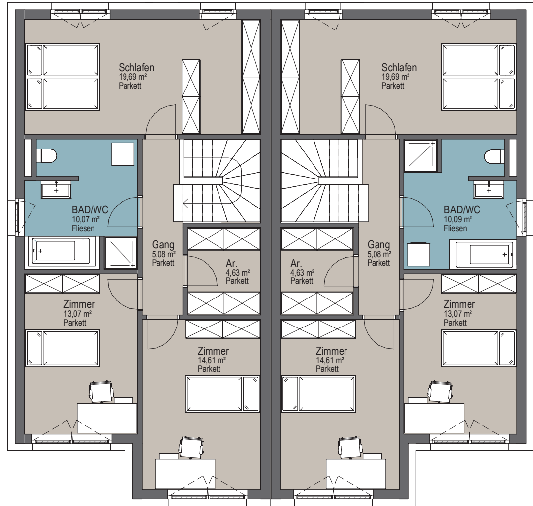
OBERGESCHOSS
